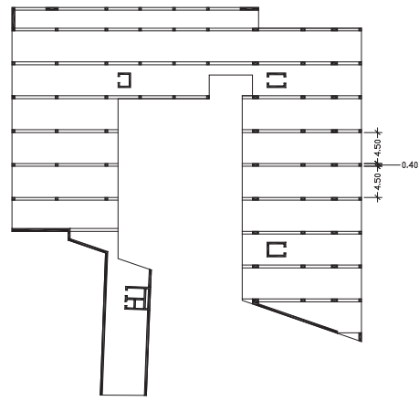
ΒΑΣΙΚΟΣ ΚΑΝΑΒΟΣ ΣΚΕΛΕΤΟΥ
